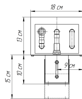
Исполнение "рв" (регулируемая высота)
