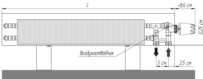
Вид для исполнения "нв" (нерегулируемая высота)
