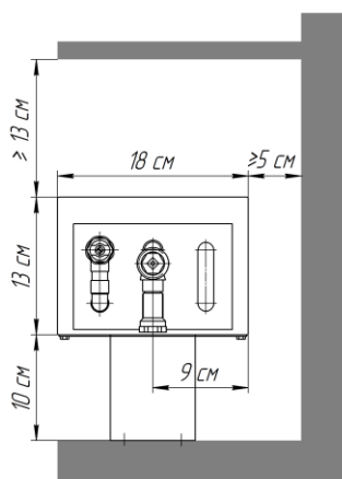
Исполнение "нв" (нерегулируемая высота)
